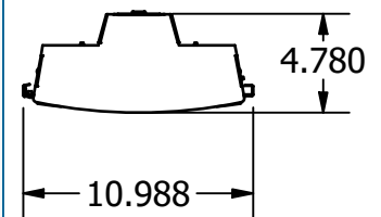
End Dimensions
